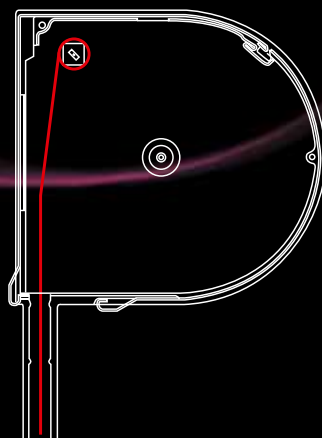
Příčný průřez oblé schránky z moskytíerou
